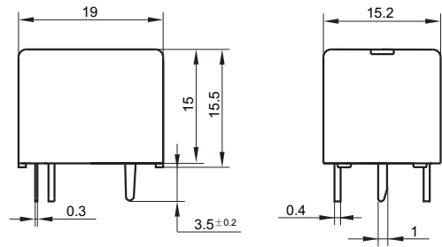
外形图
