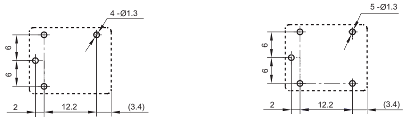
安装孔尺寸 (底视图)
