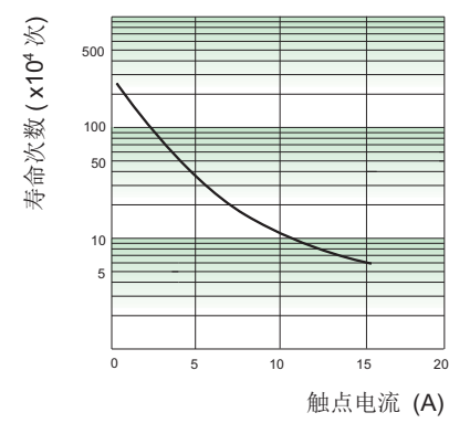
2. 电耐久性曲线
