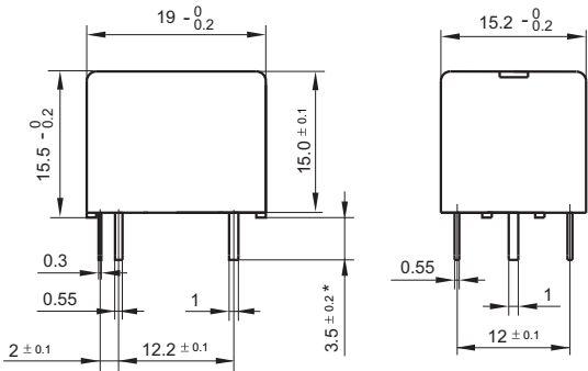
外形图（一组常开/一组转换）
