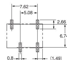
印刷基板加工尺寸(TOP VIEW) 尺寸公差为±0.1mm
