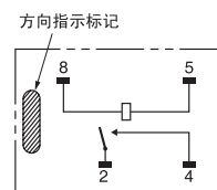
端子配置/内部连接图 (TOP VIEW)
