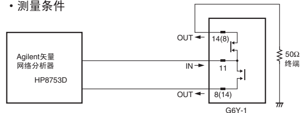
高频特性 (绝缘) *1、*2
