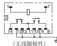
端子配置/内部接线图 (BOTTOM VIEW)
