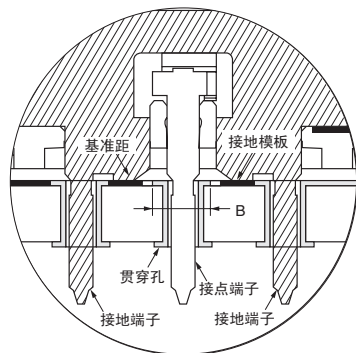
A部扩大断面图
