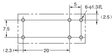
印刷基板加工尺寸 (BOTTOM VIEW)
