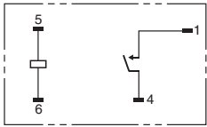
(无线圈极性)
