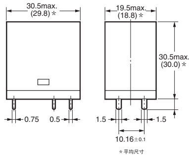
G4W-2212P-US-TV5(-Z)
