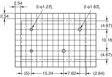
G4W-2212P-US-TV5(-Z)
