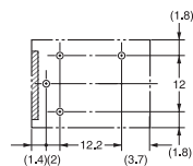
底视端子安装图
