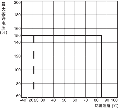
环境温度和最大容许电压
