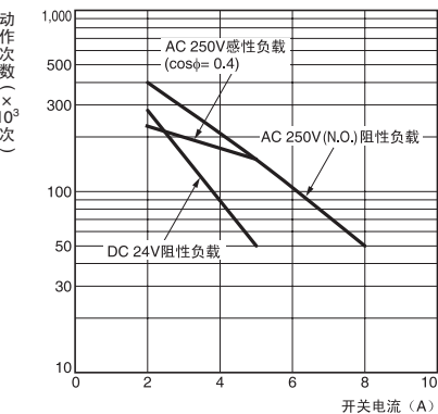
寿命曲线
