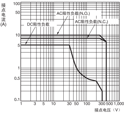
开关容量的最大值
