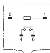
端子配置/内部连接图 (TOP VIEW)
