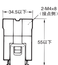
端子配置/内部连接图 (TOP VIEW)
