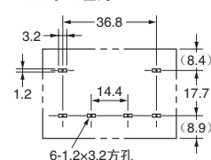
印刷基板加工尺寸 (BOTTOM VIEW)
