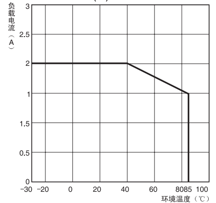
G3DZ-DZ02P(G)
