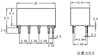
外形尺寸图
