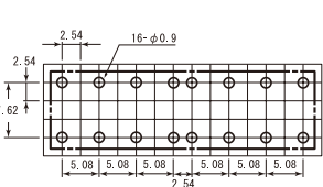
端子排列・内部接线图 (BOTTOM VIEW)
