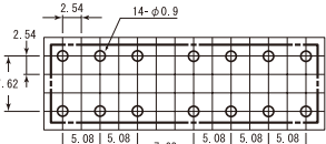
端子排列・内部接线图 (BOTTOM VIEW)
