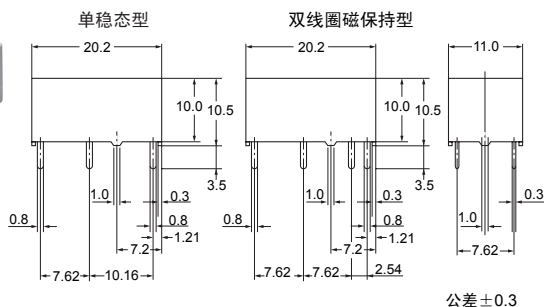
外形尺寸图
