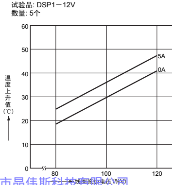
3. 一 (2) 线圈温度上升 (1a1b)
