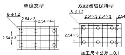
端子排列・内部接线图 (BOTTOM VIEW)
