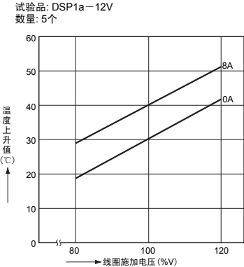
3. 一 (1) 线圈温度上升 (1a)
