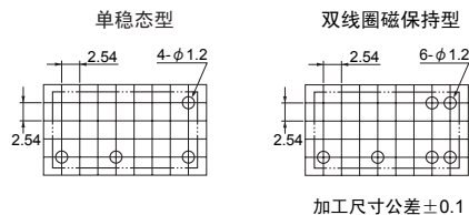
端子排列・内部接线图 (BOTTOM VIEW)
