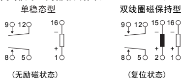
端子排列・内部接线图 (BOTTOM VIEW)
