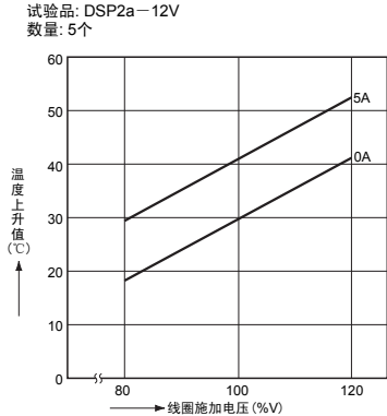
3. 一 (3) 线圈温度上升 (2a)
