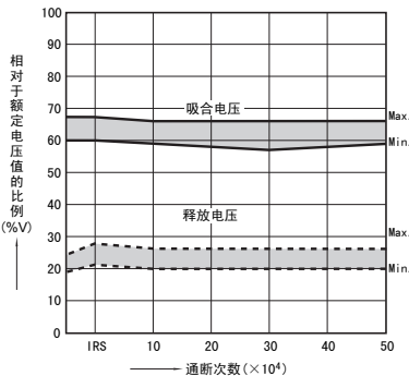
吸合·释放电压的变化(对应IRS法)
