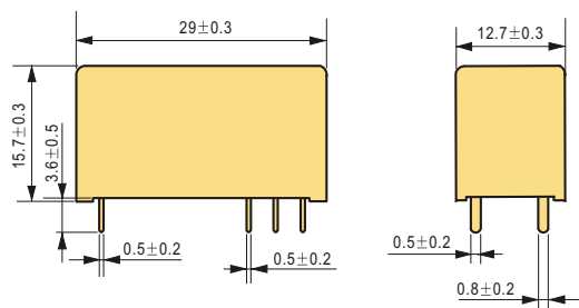
外形图
