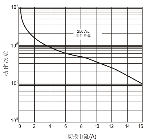
电气寿命
