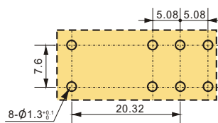
接线图
